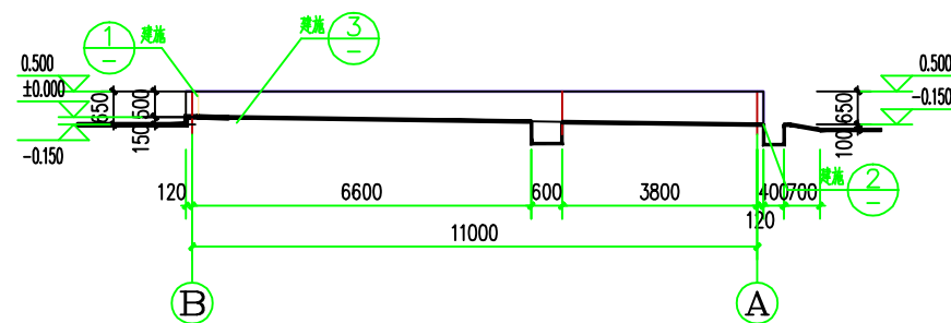
1-1剖面图 1:100
